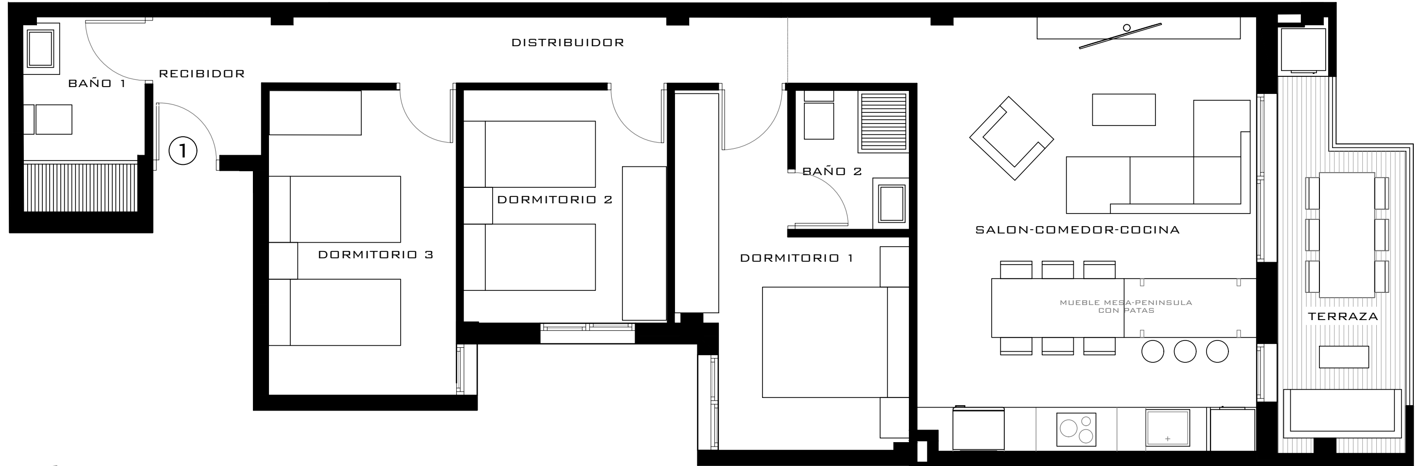
VIVIENDA TIPO 1 PLANTA 2º a 5º
